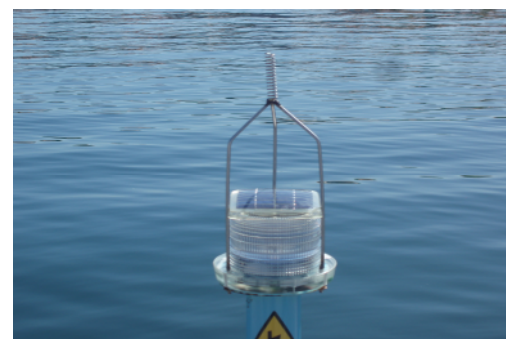
Detalle lanterna e espantapaxaros
